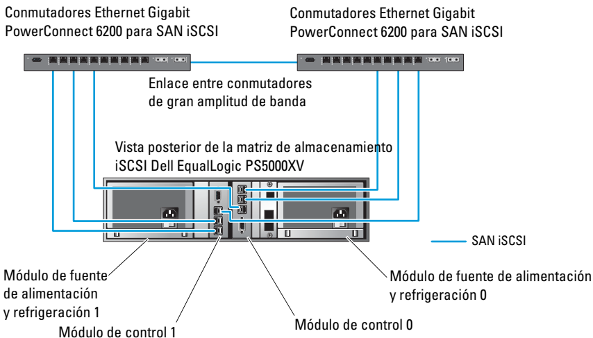
Ilustración 6-1. Configuración de red recomendada
