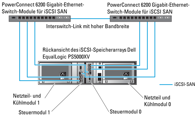
Abbildung 6-1. Empfohlene Netzwerkkonfiguration
