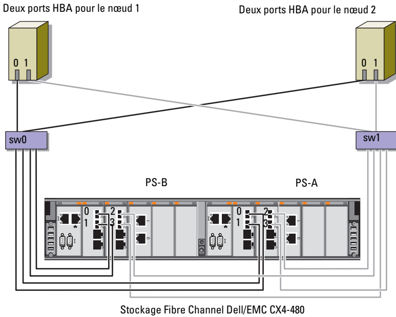
Figure 3-3. Câblage d'un cluster Fibre Channel connecté à un SAN
