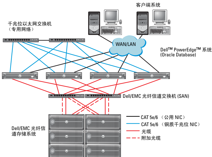
图 3-1. 光纤信道群集硬件连接
