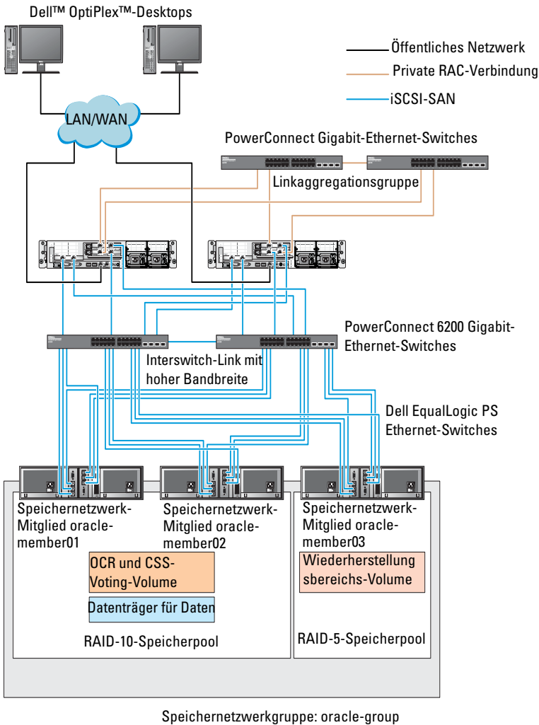
Abbildung 6-2. Oracle® RAC-Beispielkonfiguration mit drei PS5000XV-Arrays
