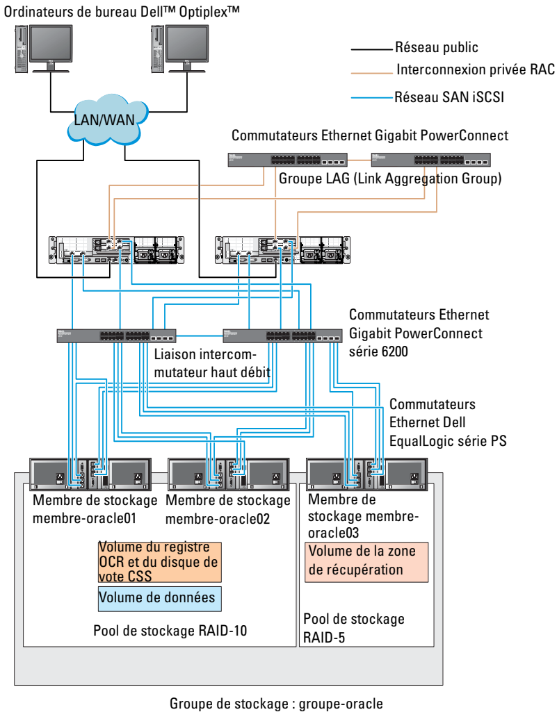
Figure 6-2. Exemple de configuration Oracle® RAC à trois baies PS5000XV
