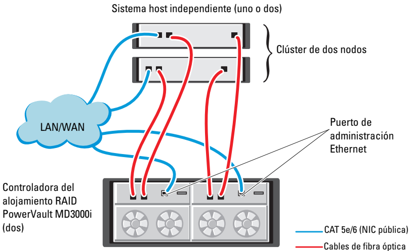
Ilustración 5-1. Cableado de los clústeres iSCSI de conexión directa
