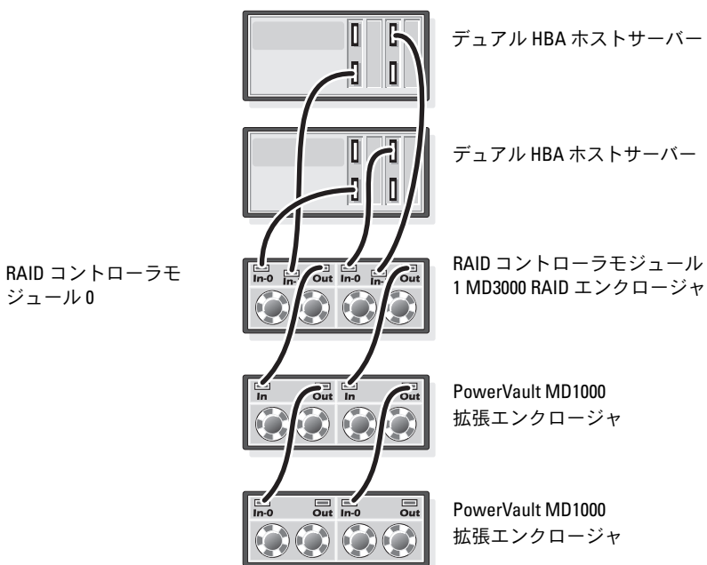
図 4-2. 直接接続 SAS クラスタのケーブル接続
