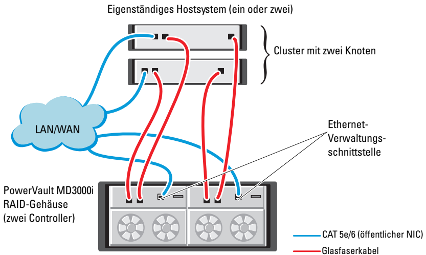
Abbildung 5-1. Direkt verbundene iSCSI-Cluster verkabeln
