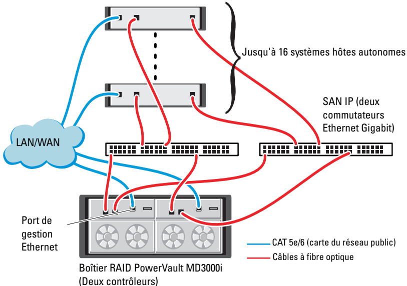
Figure 5-2. Câblage des clusters iSCSI avec liaison par commutateur
