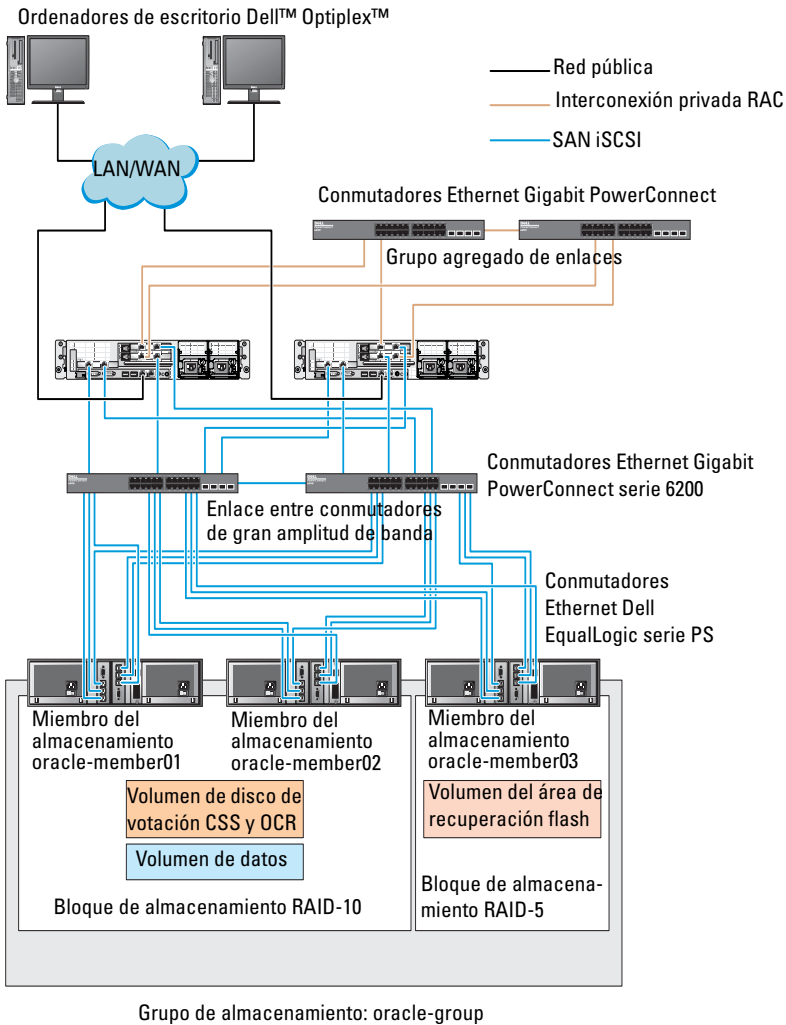
Ilustración 6-2. Configuración de Oracle® RAC de muestra con tres matrices PS5000XV
