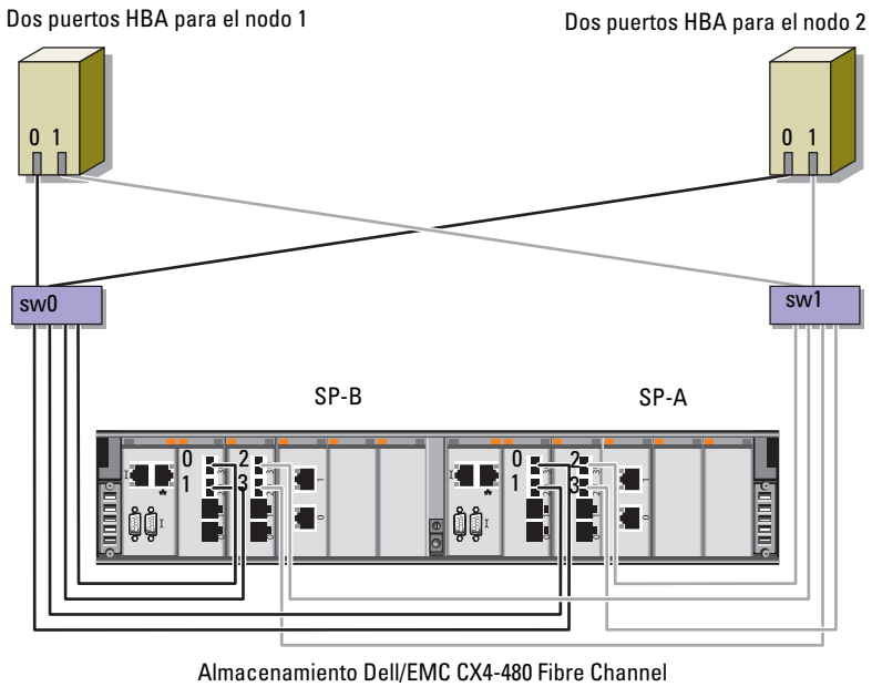
Ilustración 3-3. Cableado de un clúster Fibre Channel de conexión mediante SAN
