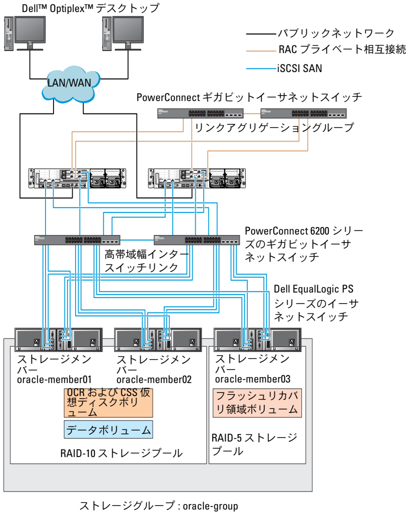
図 6-2. PS5000XV アレイ 3 つを使用した Oracle® RAC 構成例
