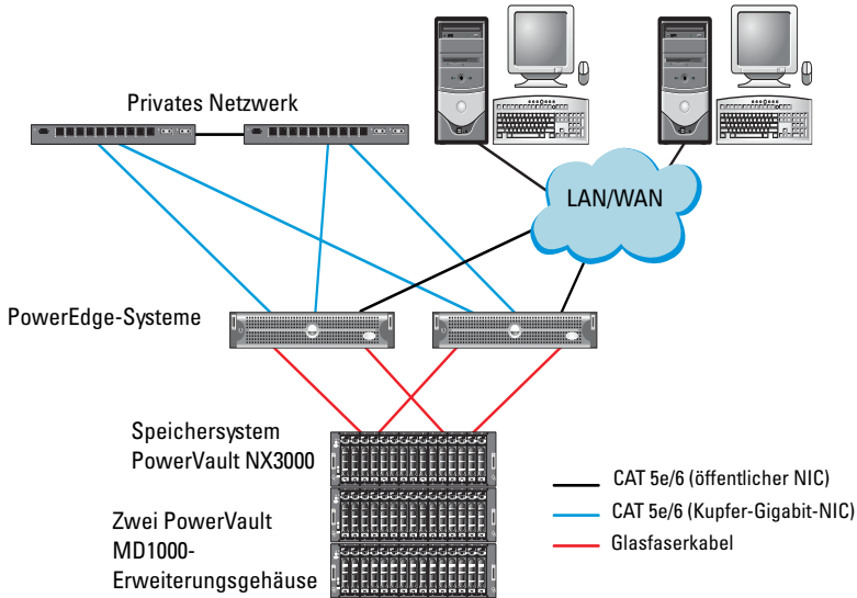
Abbildung 4-1. Verkabelung des SAS (Serial-Attached SCSI)-Clusters und des Speichergehäuses Dell PowerVault MD3000
