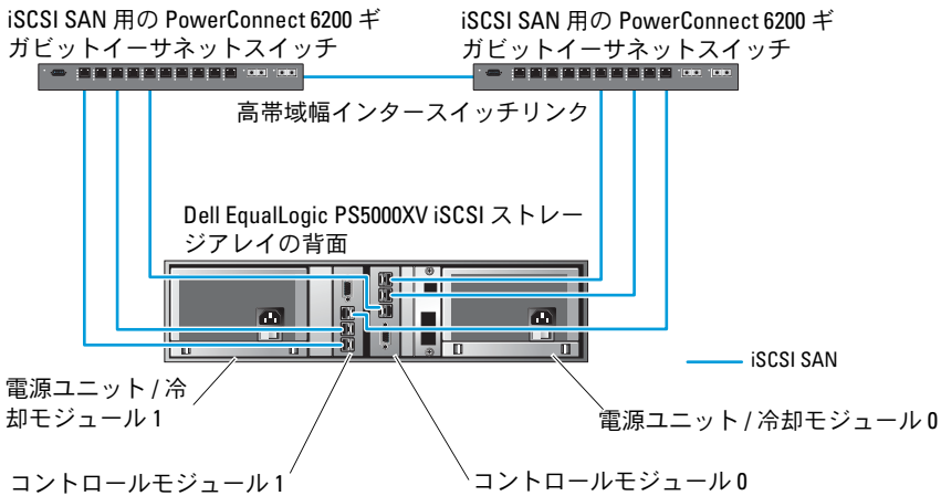
図 6-1. 推奨ネットワーク構成
