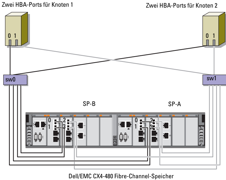
Abbildung 3-3. Verkabelung bei einem über SAN verbundenen Fibre-Channel-Cluster
