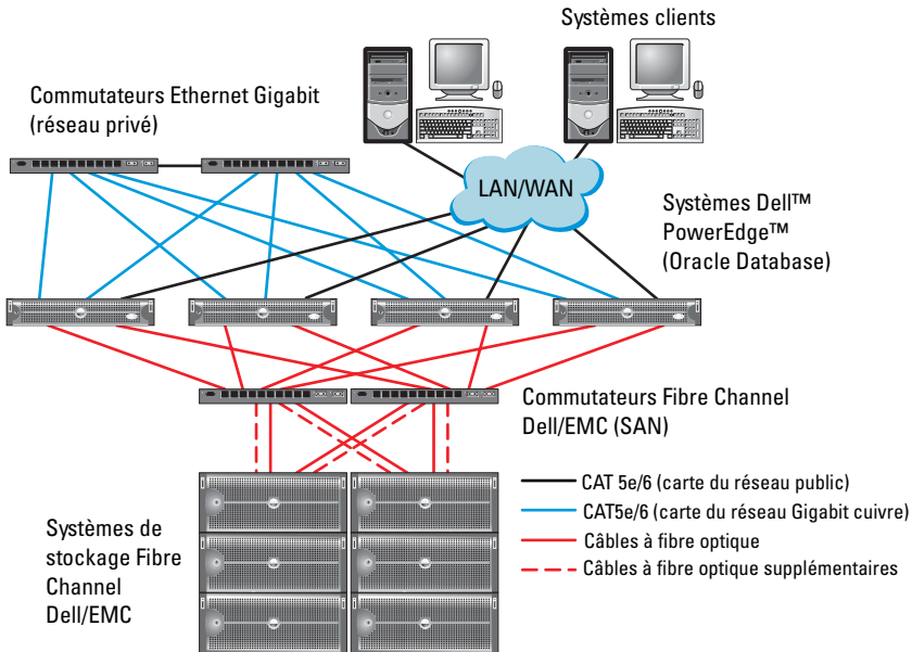
Figure 3-1. Connexions matérielles pour un cluster Fibre Channel
