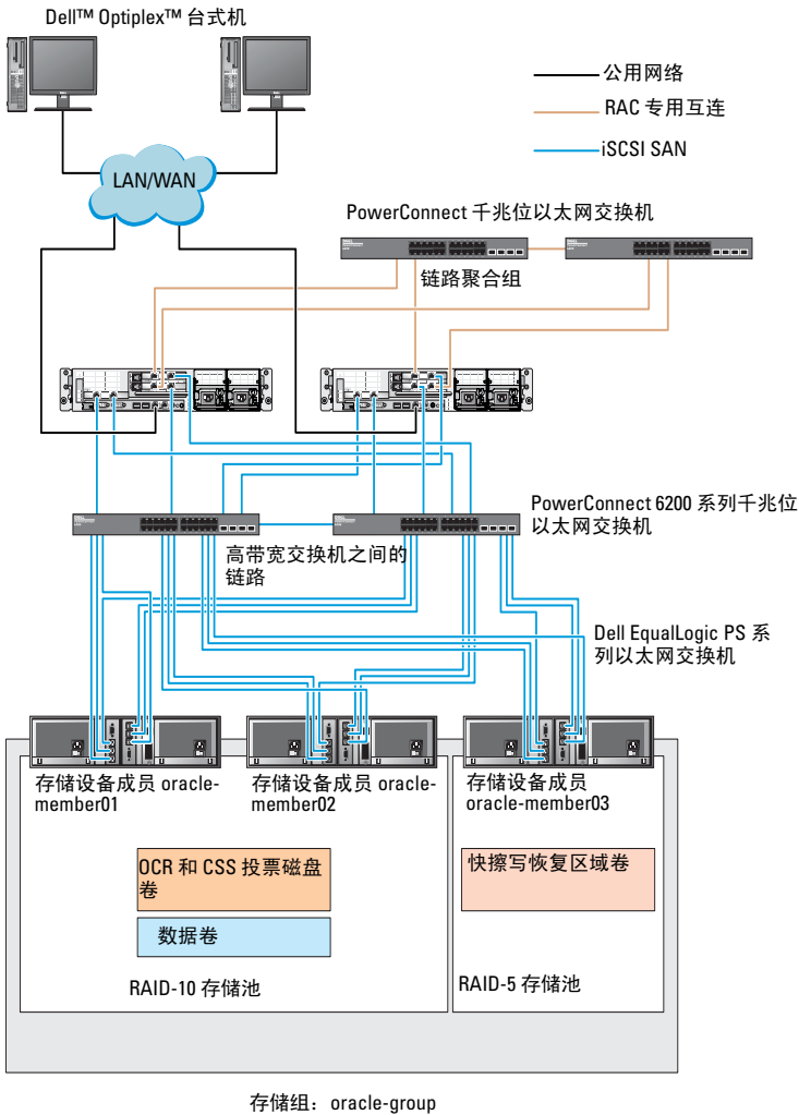
图 6-2. 带有三个 PS5000XV 阵列的示例 Oracle® RAC 配置
