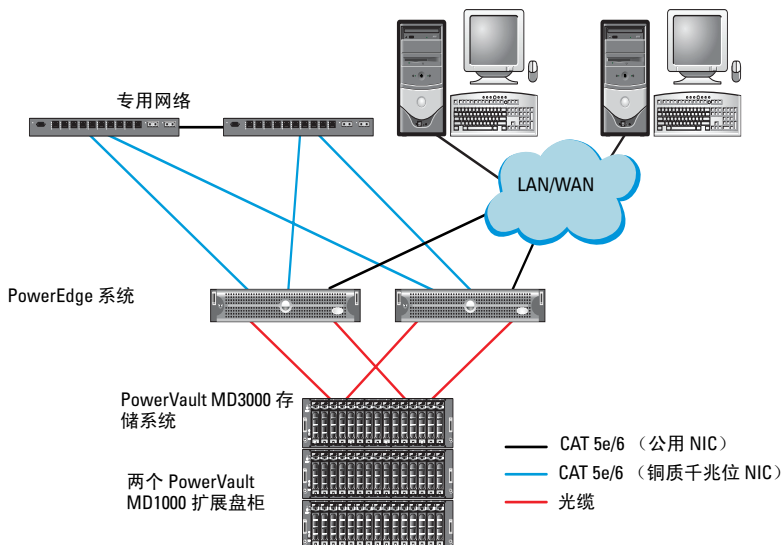
图 4-1. 串行连接的 SCSI (SAS) 群集和 Dell PowerVault MD3000 存储设备盘柜布线
