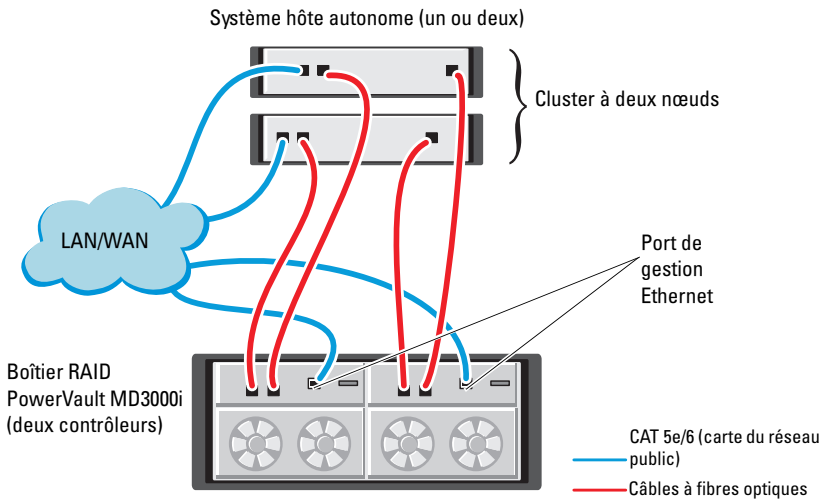
Figure 5-1. Câblage de clusters iSCSI à connexion directe
